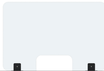
Écran en méthacrylate et verre 100/120cm Fenêtre 35x12cm La hauteur sur le table est de 67,5cm
